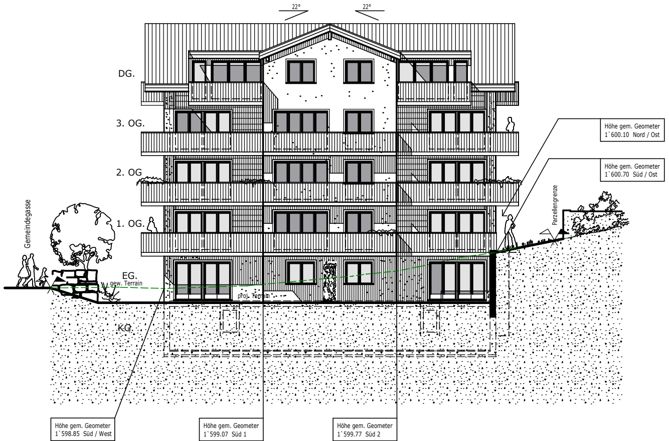
Ansicht Süd
