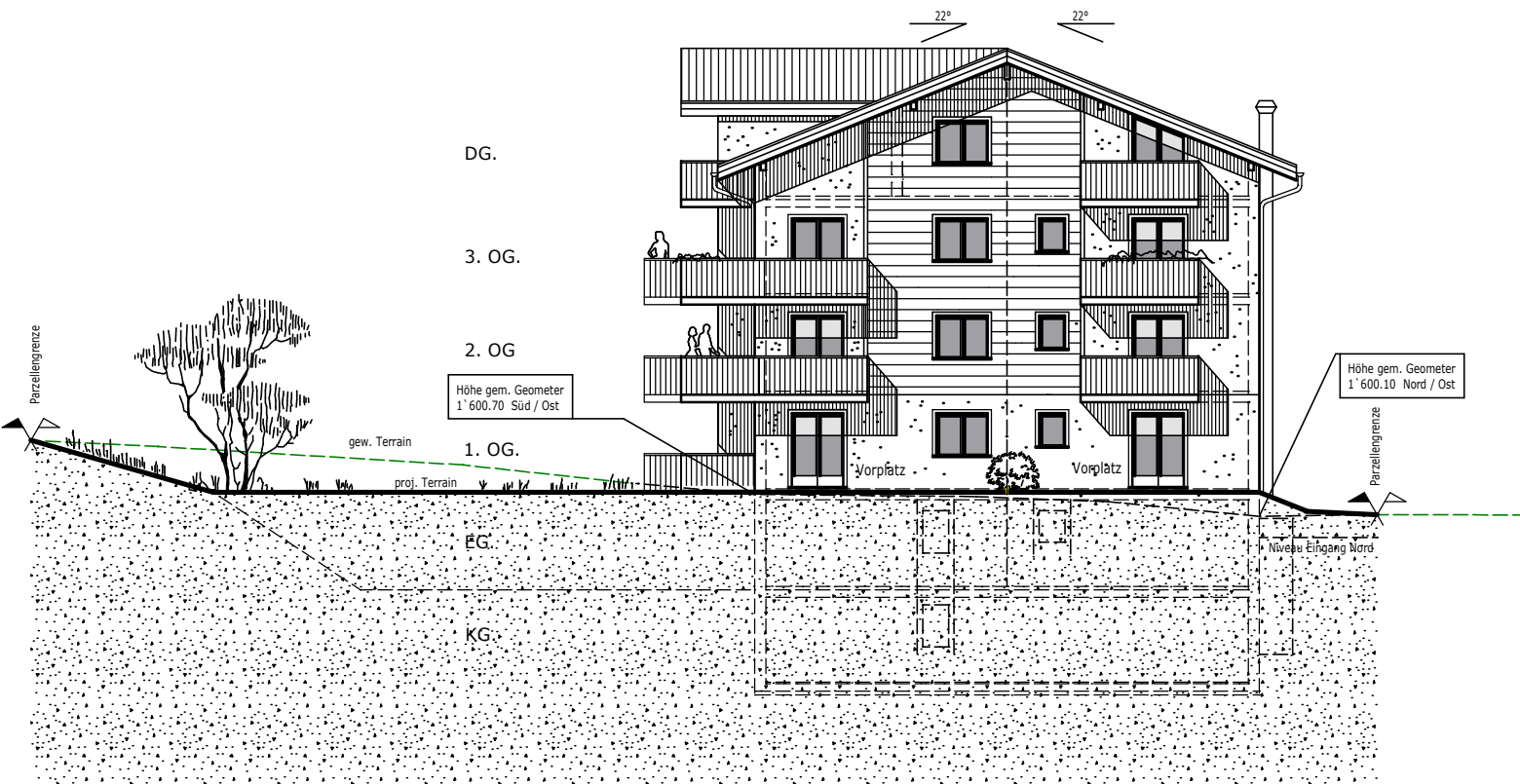
Ansicht Ost
